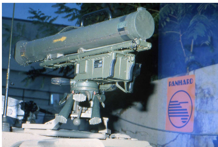
Milan-Abschusswaffe montiert auf einem Panzer (Foto: Public Domain)
