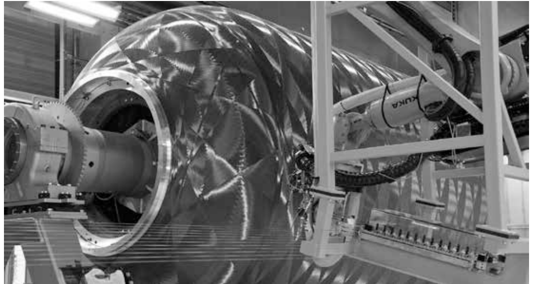
Das Boostergehäuse aus Carbonfasern für die Ariane 6 wurde beim DLR Stuttgart und Augsburg in Kooperation mit MT Aerospace entwickelt und gefertigt. Foto: 2015-07-01 (Quelle: DLR (CC-BY 3.0))
