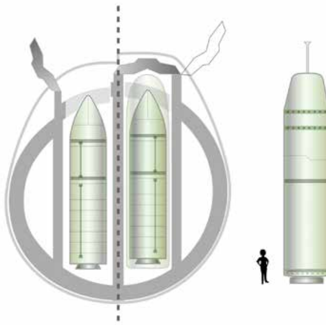
M45 und M51 Interkontinentalraketen in den Hüllen der französischen Atom-U-Boote SNLE (Typ Redoutable = schrecklich, fürchterlich, links) und SNLE-NG (Typ Triomphant, rechts), Grafik 2005-10-02 Vector version by Dake. Based on a drawing by Rama. (Quelle: Wikimedia (CC BY-SA 3.0))
